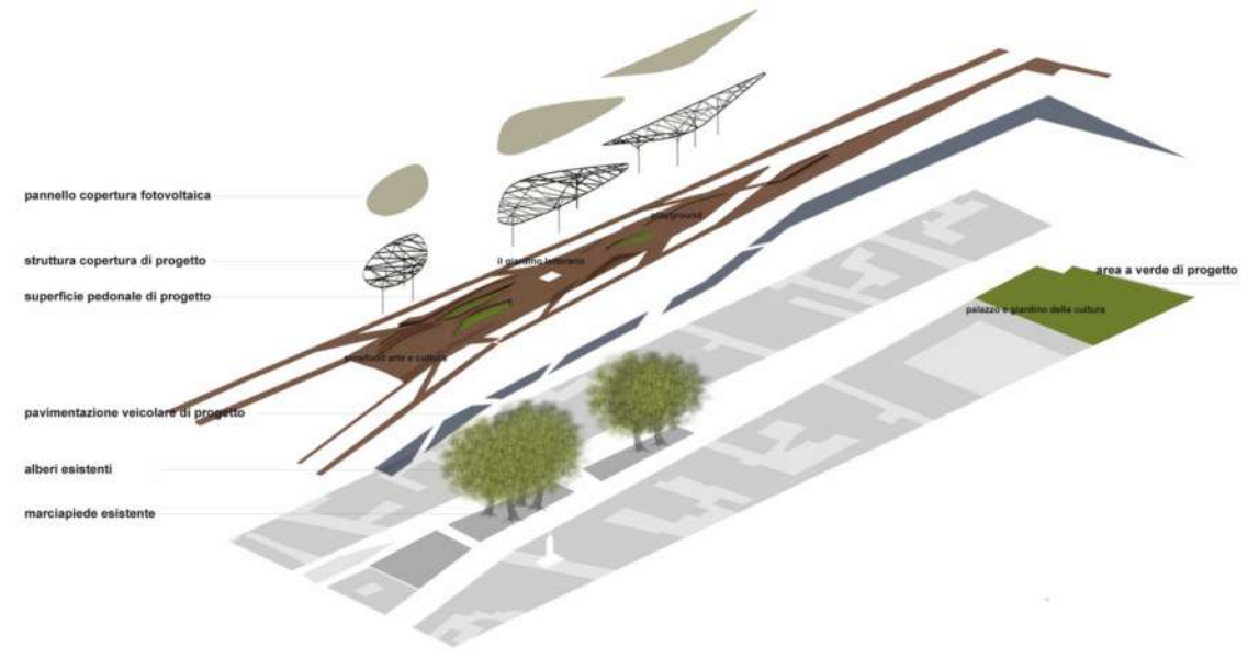
esploso assometrico dell'intervento
